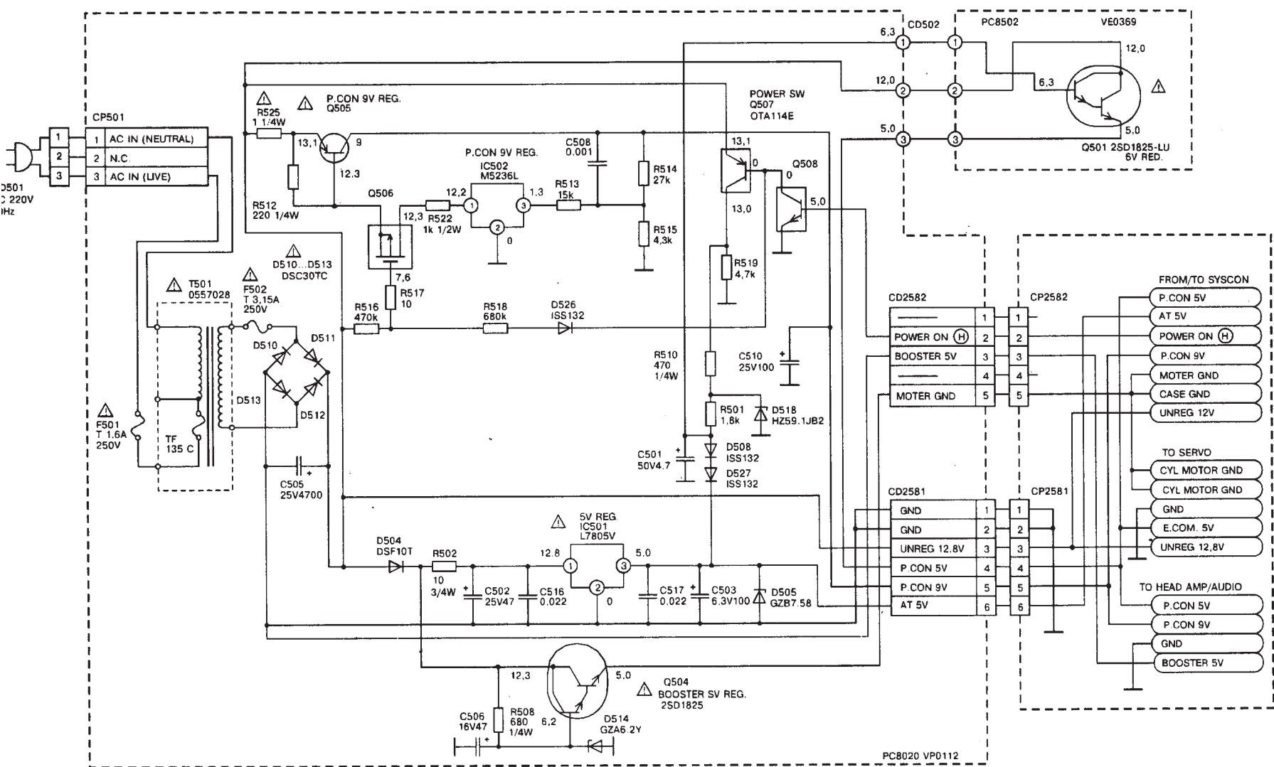
Принципиальная схема источника питания видеомэгнифона VP-300R
